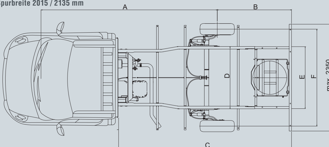
Spurbreite 2015 / 2135 mm
