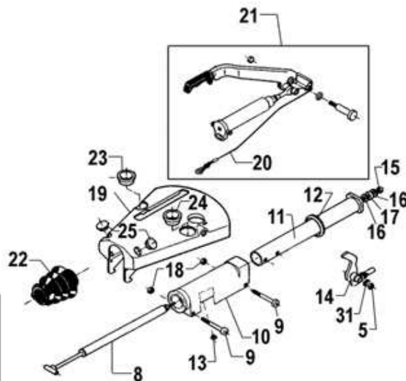
Montage Gummianschlag
