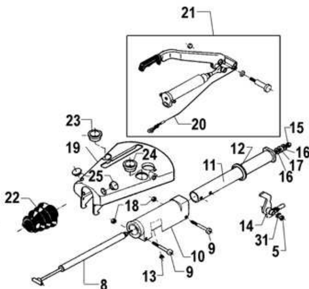
Montage Gummianschlag
