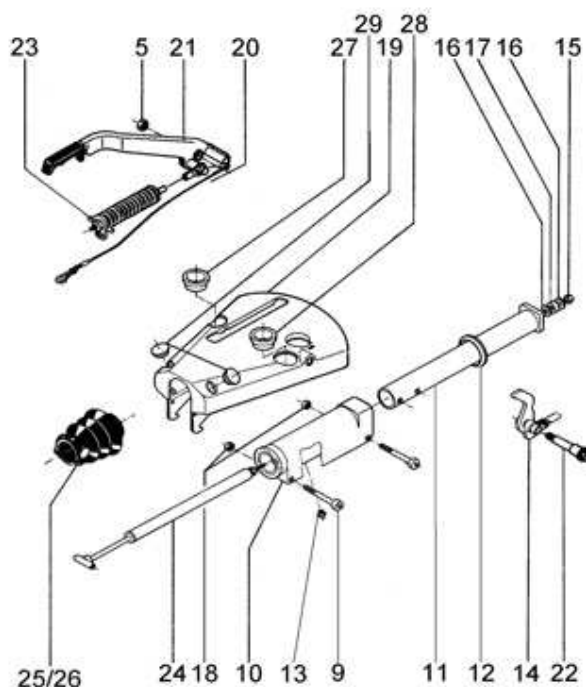
Montageteile ohne Stützradanbau
