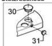
Montageteile ohne Stützradanbau
