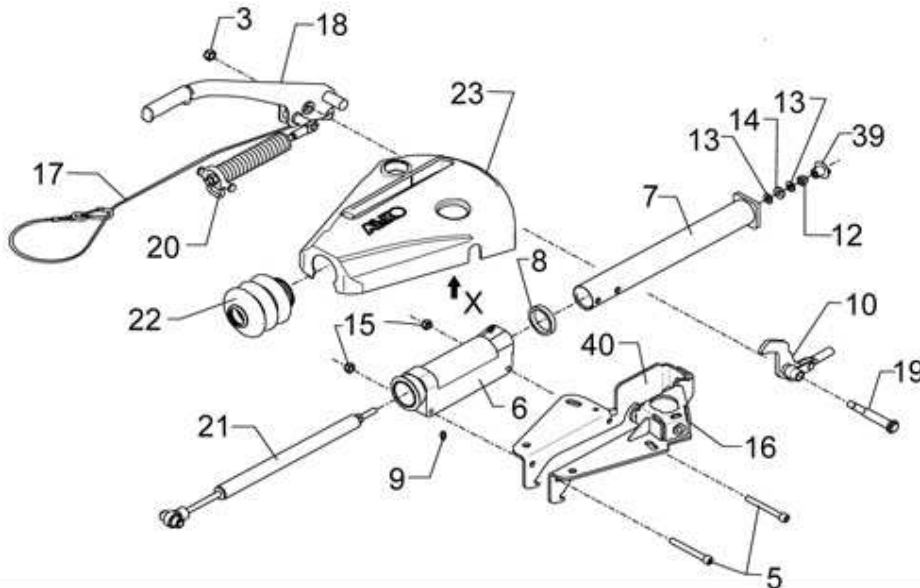
Montageteile für Stützradanbau
