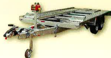
Autotransporter mit kippbarer Ladefläche, massive Ausführung (2700/3000/3500kg Gesamtgewicht)
